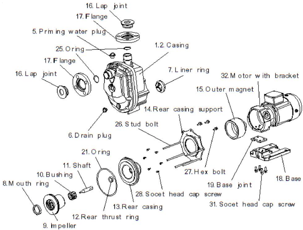
Explosionszeichnung
